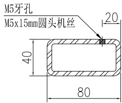
SECTION D-D
