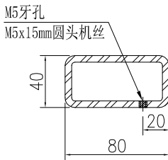
SECTION D-D
