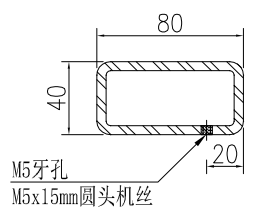
SECTION D-D
