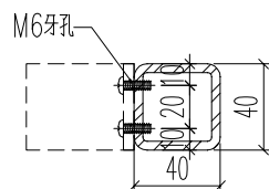
剖圖A-A
