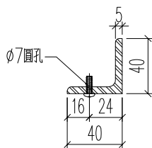
剖圖A-A
