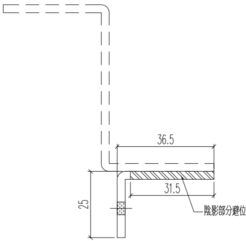
剖圖B-B
