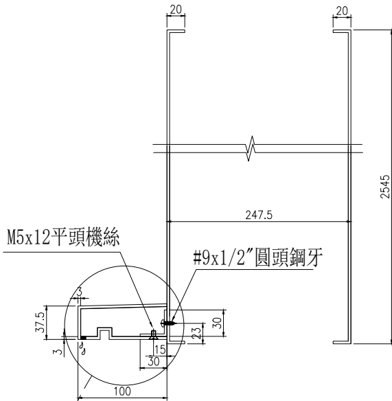
裝飾線側面安裝示意圖1
