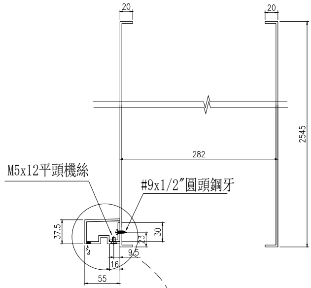
裝飾線側面安裝示意圖2
