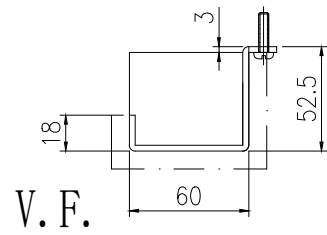
封口示意圖
