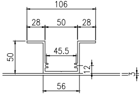
加力骨X86633
