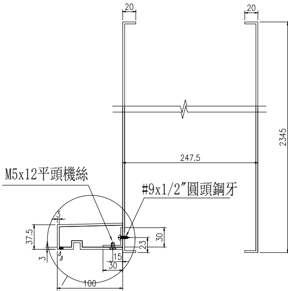
裝飾線側面安裝示意圖1
