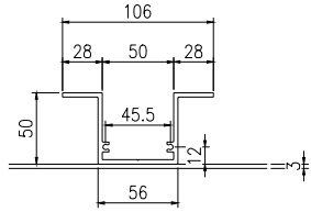
加力骨X86633
