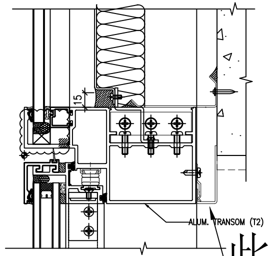
安裝示意圖
