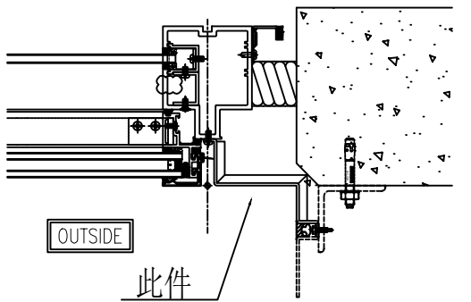
安裝示意圖
