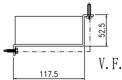
封口示意圖
