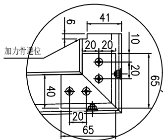
加力骨局部放大圖
