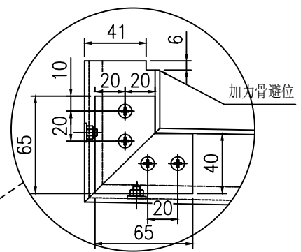
加力骨局部放大圖
