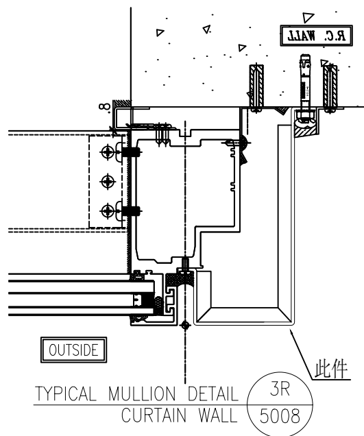
安裝示意圖
