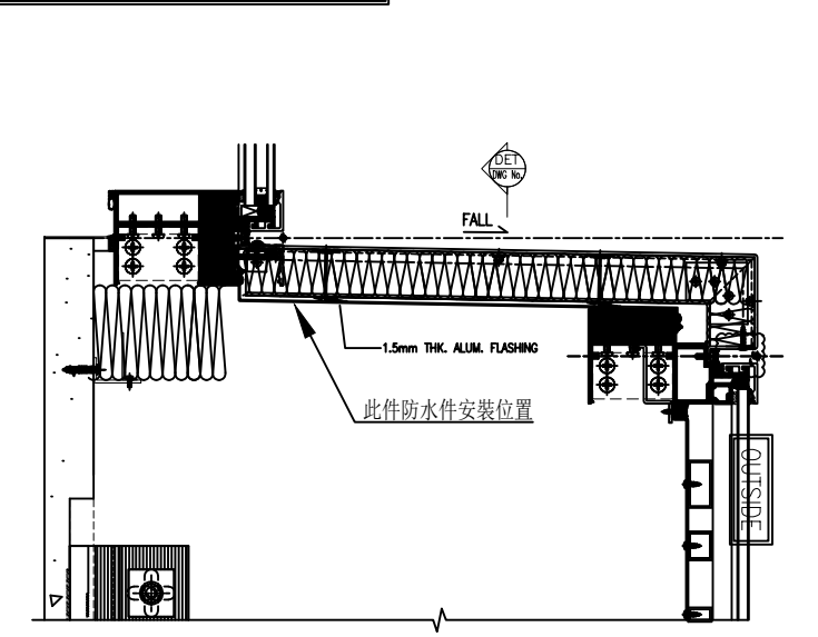
防水件安裝示意图
