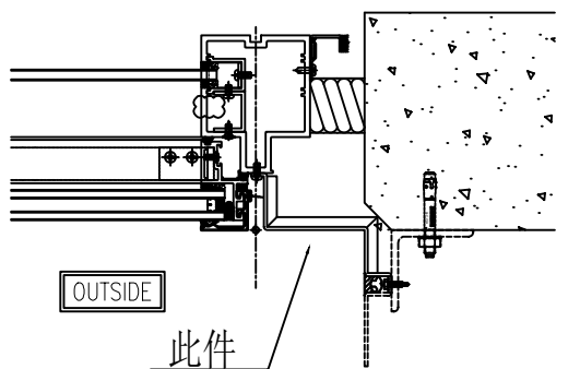
安裝示意圖
