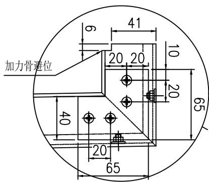
加力骨局部放大圖
