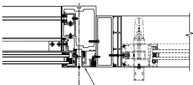
安裝示意圖
