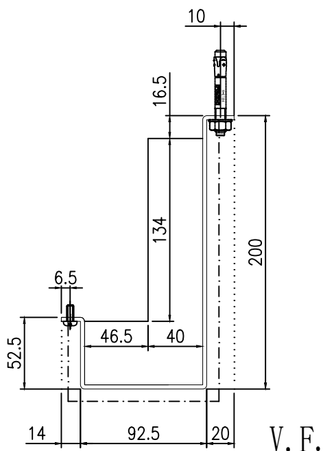
封口示意圖
