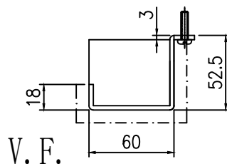
封口示意圖
