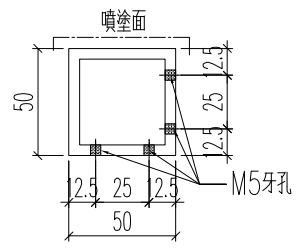
剖面A-A
