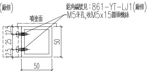
剖圖B-B
