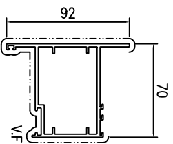
模號: X86577 名稱: FDJ門玉 合金狀態: 6063-T6 重量: 1.975KG/M V.F.: 269.7 mm
