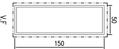
模號: I01026 名稱: 鋁通 合金狀態: 6063-T6 重量: 3.154KG/M V.F.: 400.0 mm
