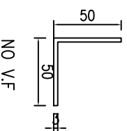
模號: L067 名稱: 50x50x3鋁角 合金狀態: 6063-T6 重量: 0.789KG/M V.F.: 0 mm
