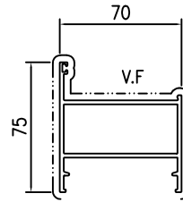
模號: X86578 名稱: FD門框企 合金狀態: 6063-T6 重量: 1.774KG/M V.F.: 239 mm
