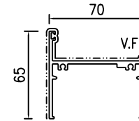
模號: X86562 名稱: FD門框底 合金狀態: 6063-T6 重量: 1.293KG/M V.F.: 249 mm
