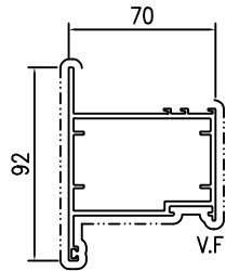
模號: X86577 名稱: FD門頂 合金狀態: 6063-T6 重量: 1.975KG/M V.F.: 269.7 mm
