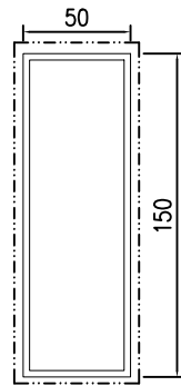
V.F. 模號: I01026 名稱: 鋁通 合金狀態: 6063-T6 重量: 3.154KG/M V.F.: 400.0 mm
