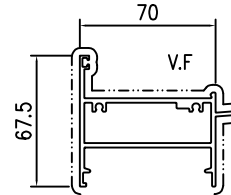
模號: X86579 名稱: FD門框頂 合金狀態: 6063-T6 重量: 1.863KG/M V.F.: 244.9 mm
