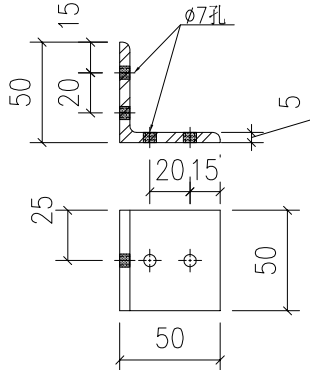
物料编号: J861-GDT1-2 规格: 50X50X5mm厚铁角 数量: 320件
