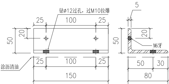
物料编号: J861-GDT1-6 规格: 80X50X5mm厚铁角 数量: 8件
