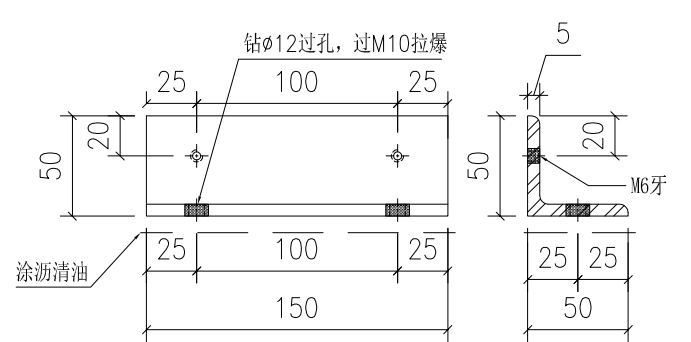
物料编号: J861-GDT1-7 规格: 50X50X5mm厚铁角 数量: 40件
