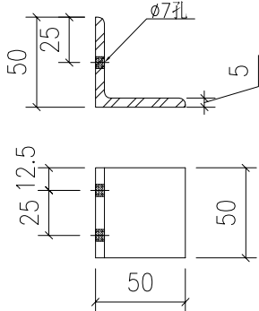
物料编号: J861-GDT1-1 规格: 50X50X5mm厚铁角 数量: 72件
