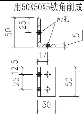
物料编号: J861-GDT1-3 规格: 50X50X5mm厚铁角 数量: 320件
