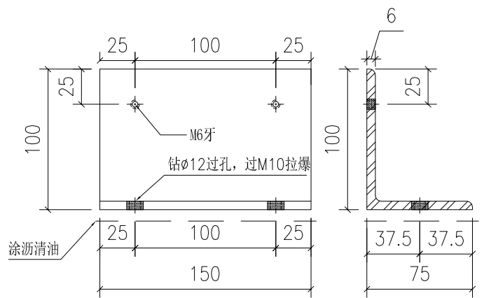
物料编号: J861-GDT1-5 规格: 100X75X6mm厚铁角 数量: 72件
