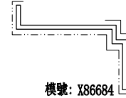
模號: X86684 名稱: 收邊 合金狀態: 6063-T6 重量: 1.168 KG/M V.F.: 216.5 mm
