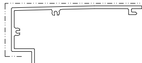
模號: X86605 名稱: 底橫冷氣位外凸 合金狀態: 6063-T6 重量: 2.113 KG/M V.F.: 307.9 mm
