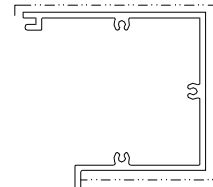
模號: X86587 名稱: 底橫室內裝飾 合金狀態: 6063-T6 重量: 2.516 KG/M V.F.: 367.1 mm
