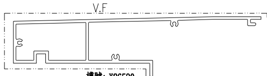
模號: X86590 名稱: 底橫室外裝飾 合金狀態: 6063-T6 重量: 4.708 KG/M V.F.: 523.8 mm
