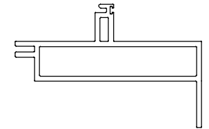
模號: X86589 名稱: 裝玻璃底橫 合金狀態: 6063-T6 重量: 4.689 KG/M V.F.: 0 mm
