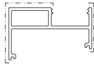
模號: X86604 名稱: 角位企冷氣位內 合金狀態: 6063-T6 重量: 2.108 KG/M V.F.: 244.6 mm
