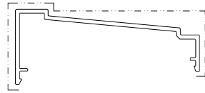
模號: X86585 名稱: 頂山 合金狀態: 6063-T6 重量: 1.954 KG/M V.F.: 293.0 mm
