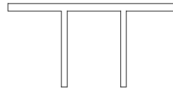
模號: X86685 名稱: 吊頂碼 合金狀態: 6063-T6 重量: 6.504 KG/M V.F.: 0 mm
