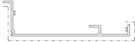
模號: X86607 名稱: 露台底 合金狀態: 6063-T6 重量: 2.777 KG/M V.F.: 418.1 mm
