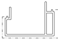
模號: X86603 名稱: 角位企冷氣位外 合金狀態: 6063-T6 重量: 2.169 KG/M V.F.: 258.4 mm
