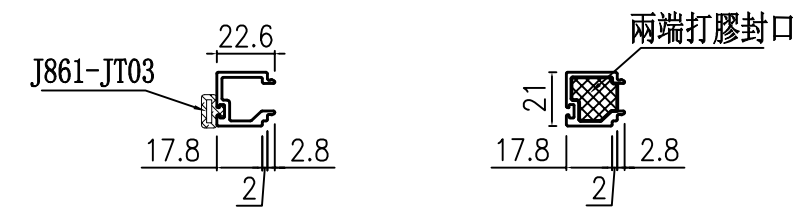
端部打膠示意圖
