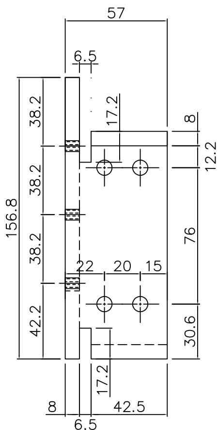
視圖 "B-B"
