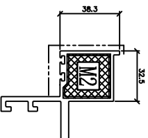
模號: X86629 名稱: 生梗企雙玻骨 合金狀態: 6063-T6 重量: 1.880 KG/M V.F.: 193 mm
