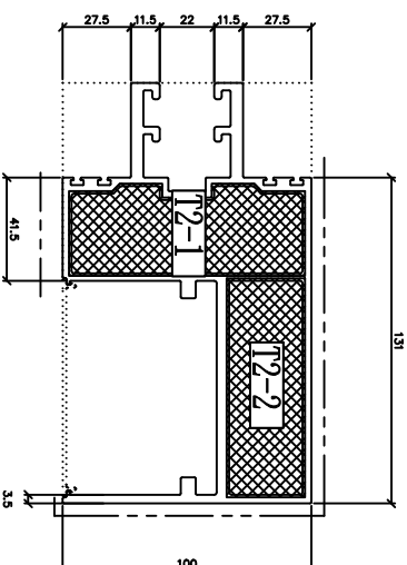
模號: X86670 名稱: 雙梗橫料 合金狀態: 6063-T6 重量: 7.189 KG/M V.F.: 531 mm
