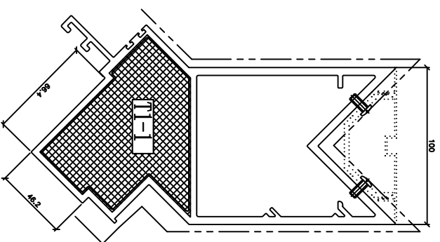
模號: X86625 名稱: 轉角企 合金狀態: 6063-T6 重量: 11.055 KG/M V.F.: 659 mm
