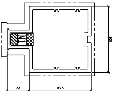
模號: X86624 名稱: 雙生企 合金狀態: 6063-T6 重量: 6.183 KG/M V.F.: 470 mm
