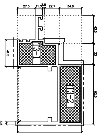
模號: X86671 名稱: 生梗橫料 合金狀態: 6063-T6 重量: 6.079 KG/M V.F.: 0.449 mm
