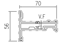
模號: X86570 名稱: 70窗扇 合金狀態: 6063-T6 重量: 1.423KG/M V.F.: 304 mm
