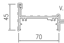
模號: X86581 名稱: 70框頂 合金狀態: 6063-T6 重量: 1.142KG/M V.F.: 213.5 mm
