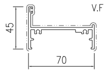
模號: X86580 名稱: 70框底 合金狀態: 6063-T6 重量: 1.085KG/M V.F.: 202.1 mm
