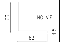
模號: L00154 名稱: 63x63x4.5鋁角 合金狀態: 6061-T6 重量: 1.481KG/M V.F.: 0 mm
