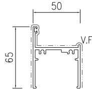
模號: X86552 名稱: 50框底 合金狀態: 6063-T6 重量: 1.163KG/M V.F.: 224 mm
