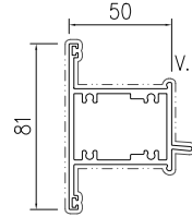
模號: X86556 名稱: 50框中橫 合金狀態: 6063-T6 重量: 1.686KG/M V.F.: 318 mm
