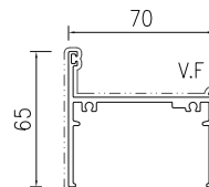
模號: X86562 名稱: FD門框底 合金狀態: 6063-T6 重量: 1.293KG/M V.F.: 249 mm
