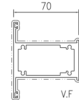
模號: X86565 名稱: 70框中企 合金狀態: 6063-T6 重量: 2.430KG/M V.F.: 339 mm
