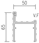
模號: X86551 名稱: 50框企 合金狀態: 6063-T6 重量: 1.023KG/M V.F.: 206 mm
