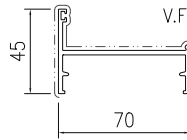
模號: X86582 名稱: 70框企 合金狀態: 6063-T6 重量: 0.939KG/M V.F.: 181.7 mm
