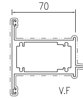
模號: X86564 名稱: 70框中橫 合金狀態: 6063-T6 重量: 2.483KG/M V.F.: 358 mm
