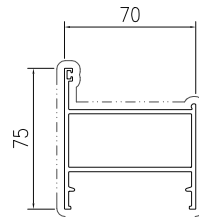
模號: X86581 名稱: 70框頂 合金狀態: 6063-T6 重量: 1.142KG/M V.F.: 213.5 mm
