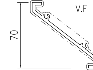
模號: X86573 名稱: 70百叶片 合金狀態: 6063-T6 重量: 1.04 KG/M V.F.: 273 mm
