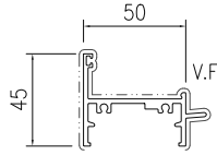
模號: X86583 名稱: 50框頂 合金狀態: 6063-T6 重量: 1.01 KG/M V.F.: 189.5 mm
