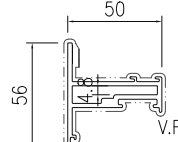
模號: X86553 名稱: 50窗扇 合金狀態: 6063-T6 重量: 1.148KG/M V.F.: 263 mm
