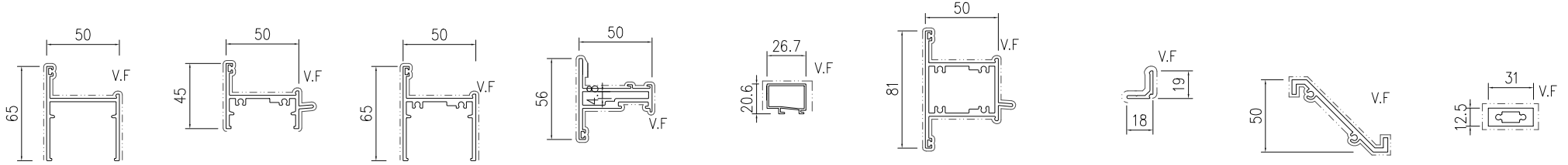
模號: X86551 名稱: 50框企 合金狀態: 6063-T6 重量: 1.023KG/M V.F.: 206 mm 模號: X86583 名稱: 50框頂 合金狀態: 6063-T6 重量: 1.01 KG/M V.F.: 189.5 mm 模號: X86552 名稱: 50框底 合金狀態: 6063-T6 重量: 1.163KG/M V.F.: 224 mm 模號: X86553 名稱: 50窗扇 合金狀態: 6063-T6 重量: 1.148KG/M V.F.: 263 mm 模號: X86554 名稱: 50扇壓綫 合金狀態: 6063-T5 重量: 0.305KG/M V.F.: 67 mm 模號: X86556 名稱: 50框中橫 合金狀態: 6063-T6 重量: 1.686KG/M V.F.: 318 mm 模號: X86043 名稱: 批水條 合金狀態: 6063-T6 重量: 0.187KG/M V.F.: 50 mm 模號: X86557 名稱: 50百葉片 合金狀態: 6063-T6 重量: 0.896KG/M V.F.: 237 mm 模號: X86576 名稱: 31x12.5鉛通 合金狀態: 6063-T6 重量: 0.734KG/M V.F.: 87 mm
