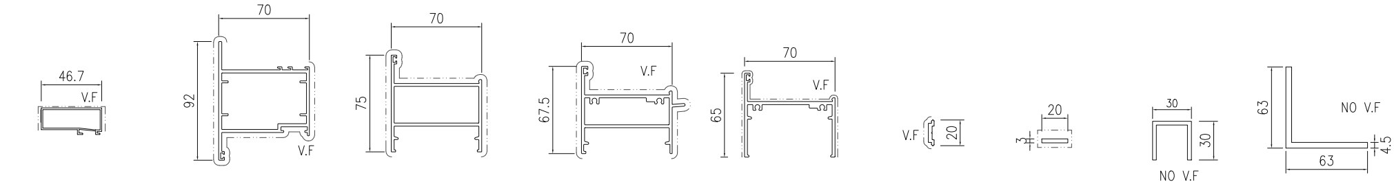
模號: X86572 名稱: 70單玻壓綫 合金狀態: 6063-T5 重量: 0.433KG/M V.F.: 91 mm 模號: X86577 名稱: FD門玉 合金狀態: 6063-T6 重量: 1.975KG/M V.F.: 269.7 mm 模號: X86578 名稱: FD門框企 合金狀態: 6063-T6 重量: 1.774KG/M V.F.: 239 mm 模號: X86579 名稱: FD門框頂 合金狀態: 6063-T6 重量: 1.863KG/M V.F.: 244.9 mm 模號: X86562 名稱: FD門框底 合金狀態: 6063-T6 重量: 1.293KG/M V.F.: 249 mm 模號: X86575 名稱: 歐標槽拉巴 合金狀態: 6063-T5 重量: 0.128KG/M V.F.: 30 mm 模號: B1502 名稱: 3x20鋁條 合金狀態: 6063-T5 重量: 0.161KG/M V.F.: 46 mm 模號: M00041 名稱: 30x30x3鋁槽 合金狀態: 6063-T6 重量: 0.68 KG/M V.F.: 0 mm 模號: L00154 名稱: 63x63x4.5鋁角 合金狀態: 6061-T6 重量: 1.481KG/M V.F.: 0 mm
