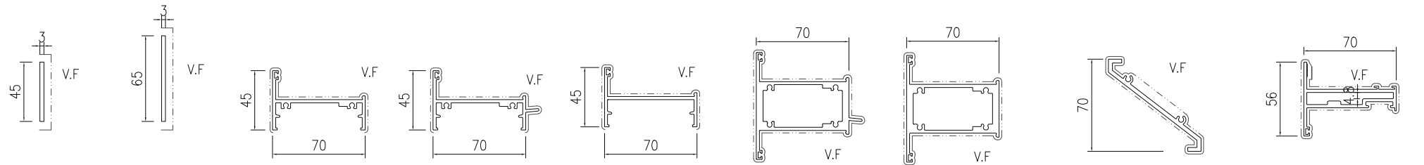
模號: B09506 名稱: 3x45鋁條 合金狀態: 6063-T5 重量: 0.4 KG/M V.F.: 51 mm 模號: B09581 名稱: 3x65鋁條 合金狀態: 6063-T5 重量: 0.529KG/M V.F.: 71 mm 模號: X86580 名稱: 70框底 合金狀態: 6063-T6 重量: 1.085KG/M V.F.: 202.1 mm 模號: X86581 名稱: 70框頂 合金狀態: 6063-T6 重量: 1.142KG/M V.F.: 213.5 mm 模號: X86582 名稱: 70框企 合金狀態: 6063-T6 重量: 0.939KG/M V.F.: 181.7 mm 模號: X86564 名稱: 70框中橫 合金狀態: 6063-T6 重量: 2.483KG/M V.F.: 358 mm 模號: X86565 名稱: 70框中企 合金狀態: 6063-T6 重量: 2.430KG/M V.F.: 339 mm 模號: X86573 名稱: 70百葉片 合金狀態: 6063-T6 重量: 1.04 KG/M V.F.: 273 mm 模號: X86570 名稱: 70窗扇 合金狀態: 6063-T6 重量: 1.423KG/M V.F.: 304 mm
