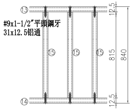
窗护栏 节点
