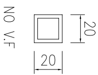
模號: N00332 名稱: 20x20x2.5方管 合金狀態: 6063-T5 重量: 0.512KG/M V.F.: 0 mm
