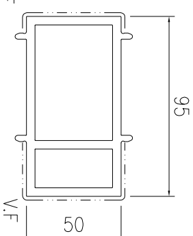
模號: X86566 名稱: 70夾通 合金狀態: 6063-T6 重量: 4.012KG/M V.F.: 201 mm
