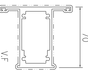
模號: X86565 名稱: 70框中企 合金狀態: 6063-T6 重量: 2.430KG/M V.F.: 339 mm
