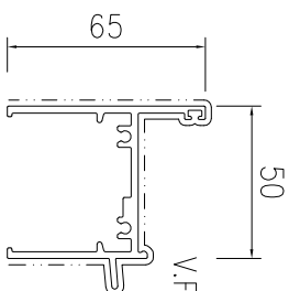
模號: X86555 名稱: 50框頂 合金狀態: 6063-T6 重量: 1.217KG/M V.F.: 236 mm
