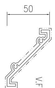
模號: X86557 名稱: 50百叶片 合金狀態: 6063-T6 重量: 0.896KG/M V.F.: 237 mm
