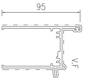
模號: X86560 名稱: 50高脚框頂 合金狀態: 6063-T6 重量: 1.591KG/M V.F.: 308 mm
