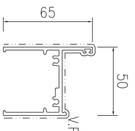
模號: X86552 名稱: 50框底 合金狀態: 6063-T6 重量: 1.163KG/M V.F.: 224 mm
