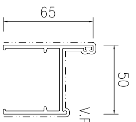
模號: X86551 名稱: 50框企 合金狀態: 6063-T6 重量: 1.023KG/M V.F.: 206 mm
