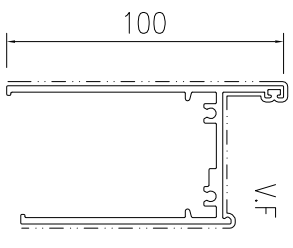
模號: X86558 名稱: 50高脚框底 合金狀態: 6063-T6 重量: 1.569KG/M V.F.: 302 mm
