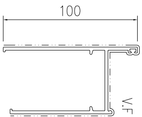
模號: X86559 名稱: 50高脚框企 合金狀態: 6063-T6 重量: 1.428KG/M V.F.: 284 mm
