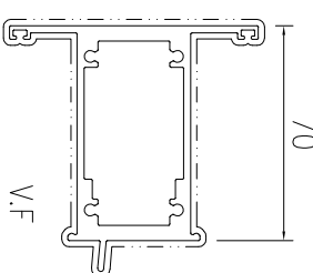
模號: X86564 名稱: 70框中橫 合金狀態: 6063-T6 重量: 2.483KG/M V.F.: 358 mm
