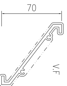
模號: X86573 名稱: 70百叶片 合金狀態: 6063-T6 重量: 1.04 KG/M V.F.: 273 mm
