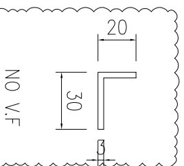
模號: N00 名稱: 63x3鋁角 合金狀態: 6063-T5 重量: 0.413KG/M V.F.: 0 mm
