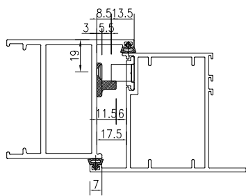
锁点与夹巴放样示意图
