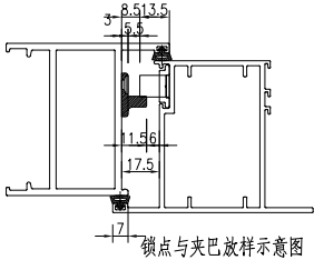
锁点与夹巴放样示意图
