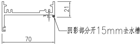
SECTION A-A
