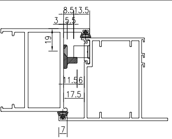
鎖點與夾巴放樣示意圖
