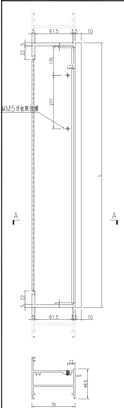
SECTION A-A
