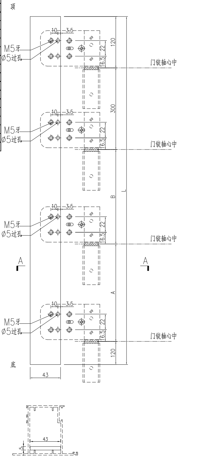
SECTION A-A
