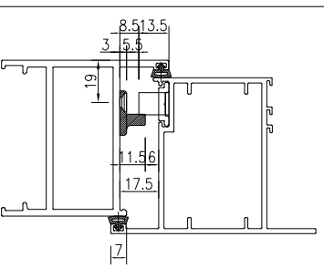
锁点与夹巴放样示意图
