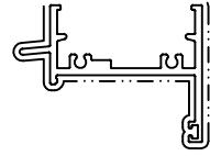
模號: X86386 名稱: 50生頂橫 合金狀態: 6063-T6 重量: 0.971KG/M V.F.: 171.3 mm
