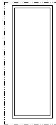
模號: JMFG0046 名稱: 140X50X3鋁通 合金狀態: 6063-T6 重量: 3.231KG/M V.F.: 380 mm
