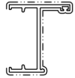
模號: X86385 名稱: 50生邊企 合金狀態: 6063-T6 重量: 0.772KG/M V.F.: 165.3 mm
