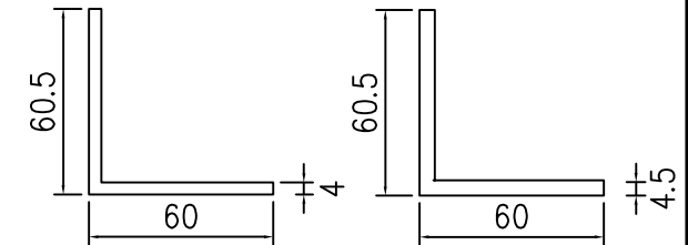
模號: JM1069 名稱: 50窗鋁角 合金狀態: 6061-T6 重量: 1.200KG/M V.F.: 0 mm
