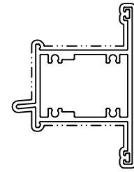
模號: X86204 名稱: 50滴水上生下生中橫 合金狀態: 6063-T6 重量: 1.891KG/M V.F.: 305.3 mm
