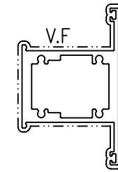
模號: X86207 名稱: 50左生右生中橫 合金狀態: 6063-T6 重量: 2.179KG/M V.F.: 299.1 mm
