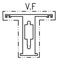
模號: X86527 名稱: 50左生右生 合金狀態: 6063-T6 重量: 1.715KG/M V.F.: 243.8 mm
