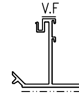
模號: X86209 名稱: 反拍線 合金狀態: 6063-T6 重量: 0.769KG/M V.F.: 52.8 mm
