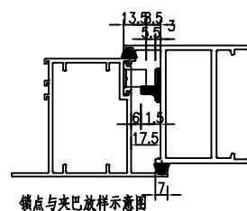
锁点与夹巴放样示意图
