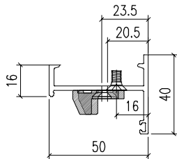
剖面A-A
