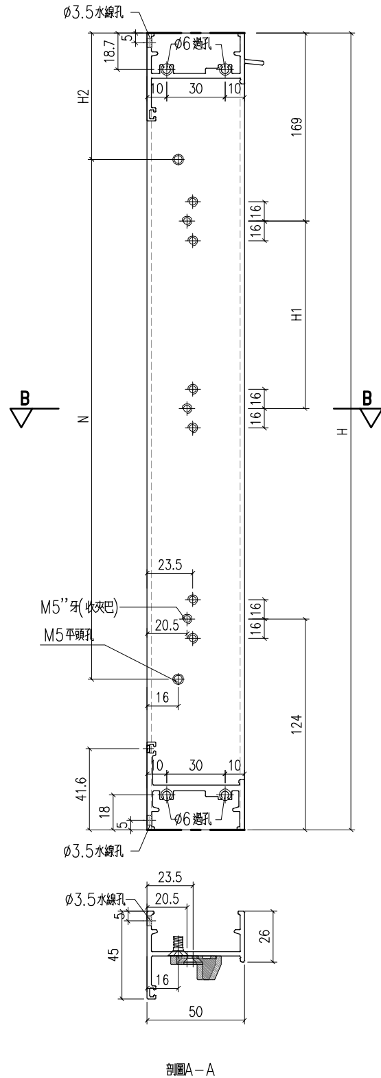
剖圖A-A
