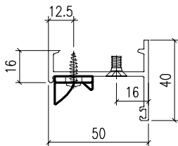
剖面A-A
