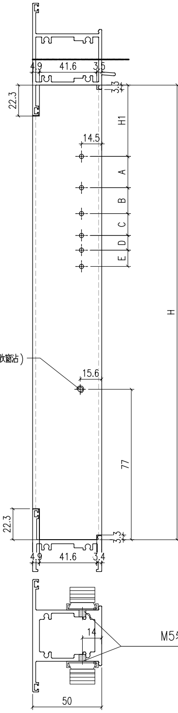
剖面A-A
