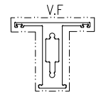
模號: X86527 名稱: 50左生右生 合金狀態: 6063-T6 重量: 1.715 KG/M V.F.: 243.8 mm
