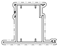
模號: X86384 名稱: FD門玉料 合金狀態: 6063-T6 重量: 2.565 KG/M V.F.: 289 mm
