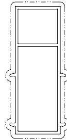
模號: X86382 名稱: 70中柱 合金狀態: 6063-T6 重量: 5.728 KG/M V.F.: 272 mm
