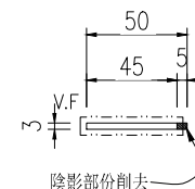
模號: BT4021 名稱: 45X3鋁巴 合金狀態: 6063-T6 重量: 0.406 KG/M V.F.: 96 mm
