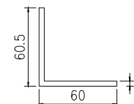
模號: JM1069 名稱: 50窗鋁角 合金狀態: 6061-T6 重量: 1.200 KG/M V.F.: 0 mm
