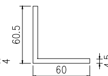
模號: JM1069A 名稱: 70窗鋁角 合金狀態: 6061-T6 重量: 1.530 KG/M V.F.: 0 mm
