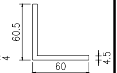
模號: JM1069A 名稱: 70窗鋁角 合金狀態: 6061-T6 重量: 1.530 KG/M V.F.: 0 mm
