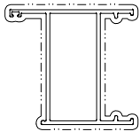
模號: X86383 名稱: 70FD門邊企料 合金狀態: 6063-T6 重量: 2.11 KG/M V.F.: 264 mm
