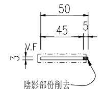
模號: BT4021 名稱: 45X3鋁巴 合金狀態: 6063-T6 重量: 0.406 KG/M V.F.: 96 mm
