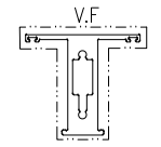
模號: X86527 名稱: 50左生右生 合金狀態: 6063-T6 重量: 1.715 KG/M V.F.: 243.8 mm
