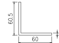
模號: JM1069 名稱: 50窗鋁角 合金狀態: 6061-T6 重量: 1.200 KG/M V.F.: 0 mm
