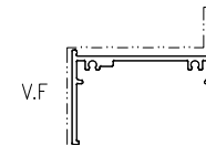
模號: X86022 名稱: 70生底橫 合金狀態: 6063-T6 重量: 1.288 KG/M V.F.: 189 mm
