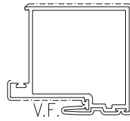
模號: X86264 名稱: 小中梗企料 合金狀態: 6063-T6 重量: 2.298 KG/M V.F.: 299 mm
