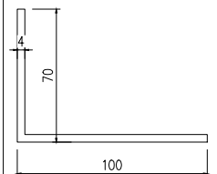
模號: N00874 名稱: 100x70x4mm厚鋁角 合金狀態: 6063-T5 重量: 1.792 KG/M V.F.: mm
