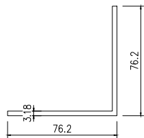
模號: L057 名稱: 76.2x76.2x3.18mm厚鋁角 合金狀態: 6063-T5 重量: 1.281 KG/M V.F.: mm
