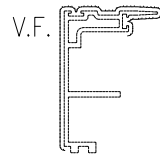
模號: X86122 名稱: 趟門勾企 合金狀態: 6063-T6 重量: 1.122 KG/M V.F.: 196 mm
