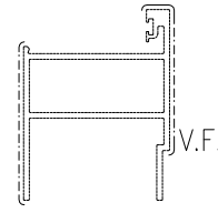
模號: X86127 名稱: 梗門企夾邊 合金狀態: 6063-T6 重量: 1.985 KG/M V.F.: 138 mm
