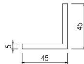
模號: H45897 名稱: 45x45x5mm厚鋁角 合金狀態: 6063-T5 重量: 1.147 KG/M V.F.: mm
