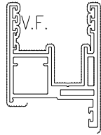
模號: X86392 名稱: 趟門玉 合金狀態: 6063-T6 重量: 2.465 KG/M V.F.: 409 mm
