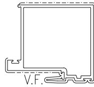
模號: X86264 名稱: 小中梗企料 合金狀態: 6063-T6 重量: 2.298 KG/M V.F.: 299 mm
