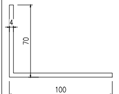
模號: N00874 名稱: 100x70x4mm厚鋁角 合金狀態: 6063-T5 重量: 1.792 KG/M V.F.: mm
