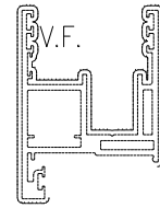
模號: X86123 名稱: 趟門玉 合金狀態: 6063-T6 重量: 2.465 KG/M V.F.: 409 mm
