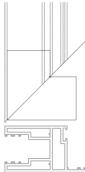
安裝示意圖
