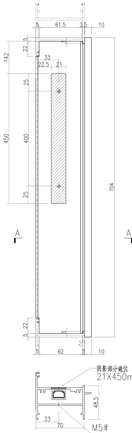
SECTION A-A
