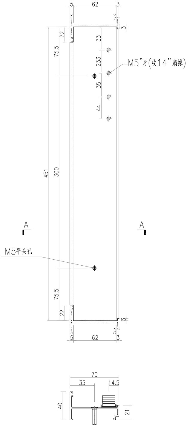
SECTION A-A
