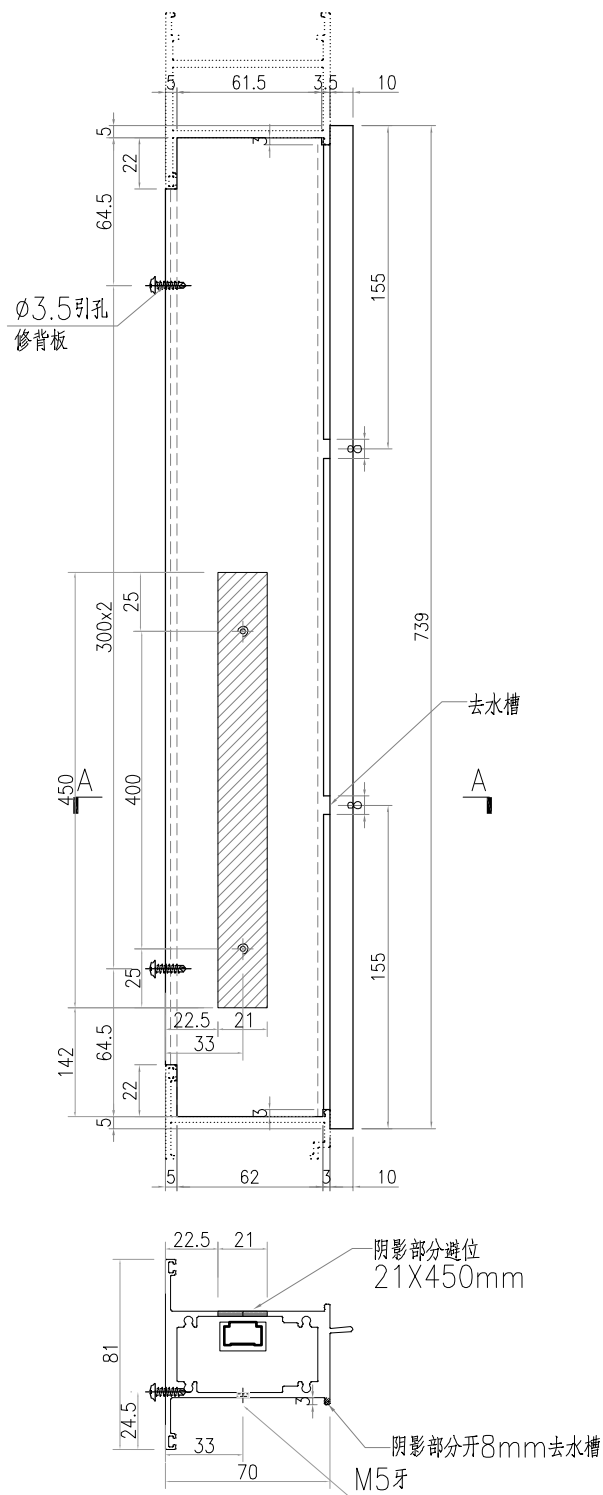
SECTION A-A
