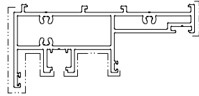
模號: X86429 名稱: 趟門頂橫料 合金狀態: 6063-T6 重量: 3.784KG/M V.F.: 376.54mm
