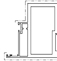
模號: X86430 名稱: 趟門梗中企 合金狀態: 6063-T6 重量: 5.705KG/M V.F.: 267.96mm
