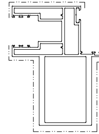
模號: X86431 名稱: 趟門玉中企 合金狀態: 6063-T6 重量: 5.858KG/M V.F.: 379.84mm
