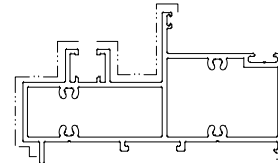
模號: X86434 名稱: 趟門底橫料 合金狀態: 6063-T6 重量: 3.864KG/M V.F.: 367.21mm
