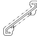
模號: X85958 名稱: 70百葉片 合金狀態: 6063-T6 重量: 1.041 KG/M V. F.: 272 mm
