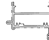
模號: X86269 名稱: 70FD門頂橫料 合金狀態: 6063-T6 重量: 1.772KG/M V.F.: 236.5 mm
