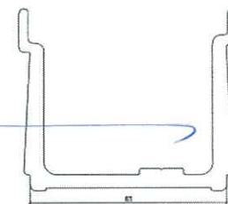
SCALE 2:1 NO V.F. 模號: X86303 名稱: 水槽套芯 合金狀態: 6061-T6 重量: 2.329 KG/M V.F.: - mm
