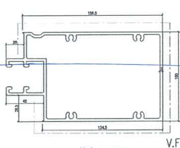
模號: X86302 名稱: 梗中橫 合金狀態: 6063-T6 重量: 5.428 KG/M V.F.: 125.4 mm
