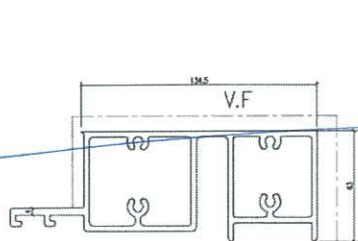
模號: X86290 名稱: 底橫 合金狀態: 6063-T6 重量: 5.134 KG/M V.F.: 381.0 mm
