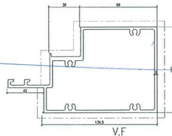
模號: X86281 名稱: 生下梗中橫 合金狀態: 6063-T6 重量: 4.926 KG/M V.F.: 489.9 mm
