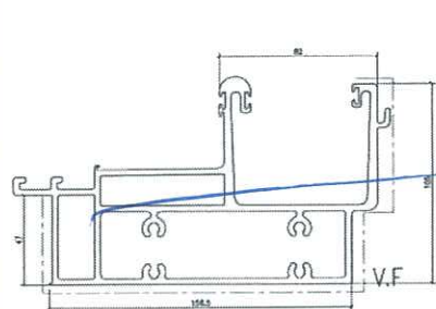
模號: X86279 名稱: 水槽橫 合金狀態: 6063-T6 重量: 7.453 KG/M V.F.: 538.0 mm
