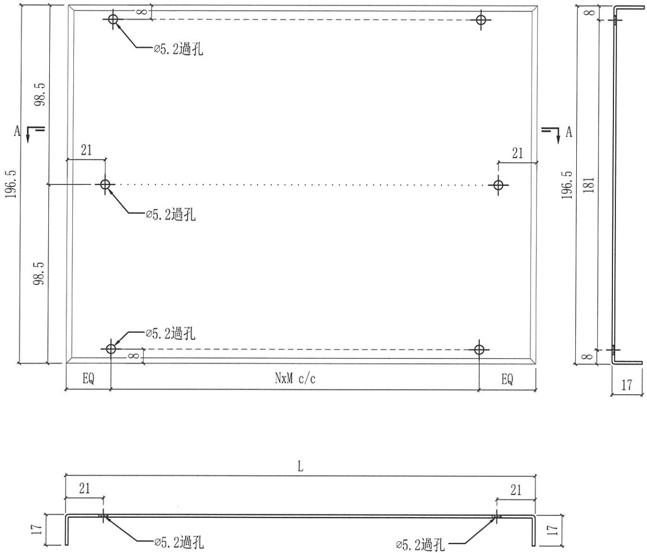
SECTION A-A
