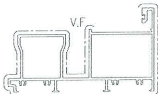
模號: X86332 名稱: 趟門頂橫 合金狀態: 6063-T5 重量: 3.74 KG/M V.F.: 488.2 mm
