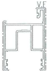
模號: X86344 名稱: 生門玉企及頂底料 合金狀態: 6063-T5 重量: 2.777 KG/M V.F.: 349.1 mm
