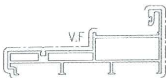
模號: X86334 名稱: 趟門梗企框 合金狀態: 6063-T5 重量: 3.107 KG/M V.F.: 363.7 mm
