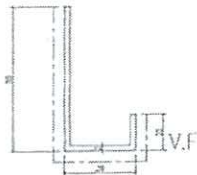
模號: X86464 名稱: 趟門降底收口 合金狀態: 6063-T5 重量: 1.081 KG/M V.F.: 139.0 mm
