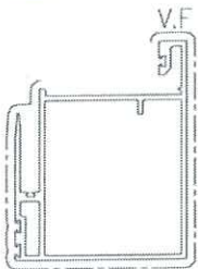
模號: X86343 名稱: 生門玉企料 合金狀態: 6063-T5 重量: 2.778 KG/M V.F.: 311.6 mm
