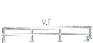
模號: X86322 名稱: 趟門生企框 合金狀態: 6063-T5 重量: 2.436 KG/M V.F.: 271.4 mm
