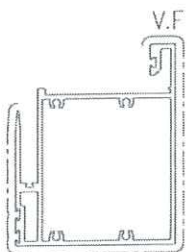
模號: X86345 名稱: 梗門玉料 合金狀態: 6063-T5 重量: 2.932 KG/M V.F.: 312.8 mm
