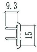
SECTION A-A
