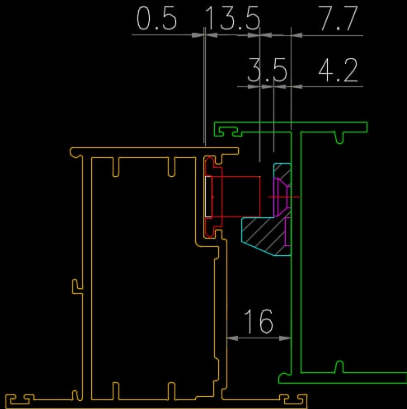
锁点与夹巴放样示意图
