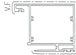
模號: X86345 名稱: 梗門玉料 合金狀態: 6063-T5 重量: 2.932 KG/M V.F.: 312.8 mm
