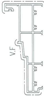
模號: X86330 名稱: 趟門底橫 合金狀態: 6063-T5 重量: 3.329 KG/M V.F.: 412.4 mm
