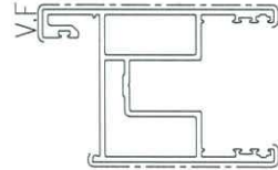
模號: X86344 名稱: 生門玉企及頂底料 合金狀態: 6063-T5 重量: 2.777 KG/M V.F.: 349.1 mm
