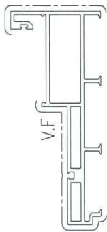
模號: X86324 名稱: 趟門梗企框 合金狀態: 6063-T5 重量: 3.107 KG/M V.F.: 363.7 mm
