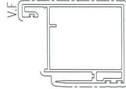
模號: X86343 名稱: 生門玉企料 合金狀態: 6063-T5 重量: 2.778 KG/M V.F.: 311.6 mm
