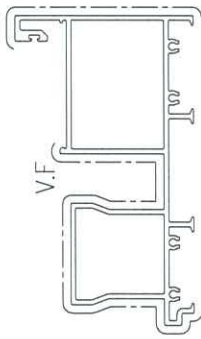
模號: X86332 名稱: 趟門頂橫 合金狀態: 6063-T5 重量: 3.74 KG/M V.F.: 488.2 mm
