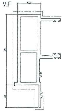
模號: X86272 名稱: 梗公企 合金狀態: 6063-T6 重量: 6.569 KG/M V.F.: 109.7 mm
