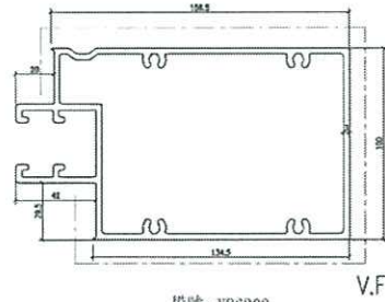
模號: X86302 名稱: 梗中橫 合金狀態: 6063-T6 重量: 5.428 KG/M V.F.: 125.1 mm
