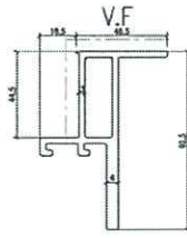
模號: X86293 名稱: GC底橫 合金狀態: 6063-T6 重量: 2.260 KG/M V.F.: 210.3 mm
