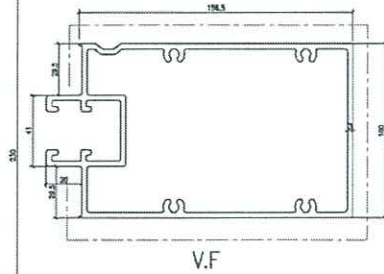
模號: X86308 名稱: Feature 中橫 合金狀態: 6063-T6 重量: 5.607 KG/M V.F.: 709.0 mm
