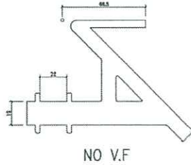
模號: X86256 名稱: 掛勾碼 合金狀態: 6061-T6 重量: 11.63 KG/M V.F.: - mm
