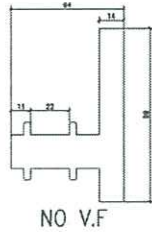
模號: X86255 名稱: 掛勾碼 合金狀態: 6061-T6 重量: 6.63 KG/M V.F.: - mm
