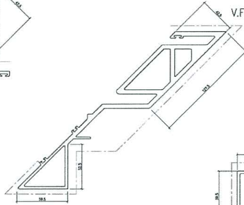
模號: X86276 名稱: 轉角生母企 合金狀態: 6063-T6 重量: 8.759 KG/M V.F.: 575.1 mm
