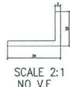
模號: X86287 名稱: 鋁板角 合金狀態: 6063-T5 重量: 0.38 KG/M V.F.: - mm
