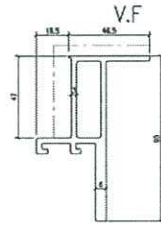
模號: X86292 名稱: GC頂橫 合金狀態: 6063-T6 重量: 2.301 KG/M V.F.: 213.3 mm
