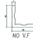
模號: X86318 名稱: 幕牆窗玉角 合金狀態: 6063-T5 重量: 1.624 KG/M V.F.: - mm
