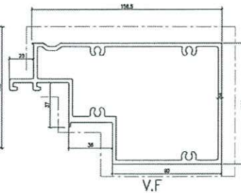
模號: X86309 名稱: 生中橫 合金狀態: 6063-T6 重量: 5.137 KG/M V.F.: 594.9 mm
