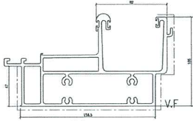
模號: X86279 名稱: 水槽橫 合金狀態: 6063-T6 重量: 7.453 KG/M V.F.: 538.0 mm
