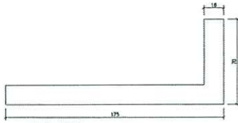
模號: X86266 名稱: 鋁碼 合金狀態: 6061-T6 重量: 9.12 KG/M V.F.: - mm
