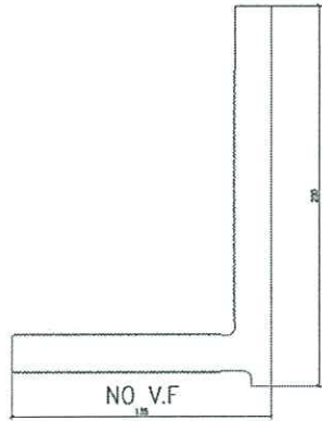
模號: X86254 名稱: 大鋁碼 合金狀態: 6061-T6 重量: 16.58 KG/M V.F.: - mm
