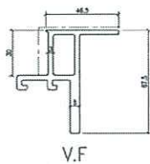
模號: X86291 名稱: GC中橫 合金狀態: 6063-T6 重量: 1.853 KG/M V.F.: 180.3 mm
