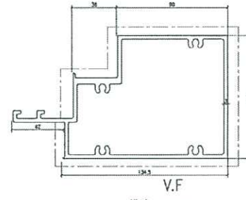
模號: X86281 名稱: 生下梗中橫 合金狀態: 6063-T6 重量: 4.926 KG/M V.F.: 489.9 mm
