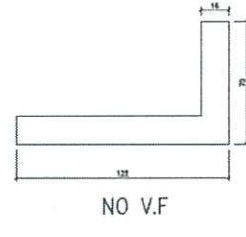
模號: X86257 名稱: 大鋁碼 合金狀態: 6061-T6 重量: 7.63 KG/M V.F.: - mm
