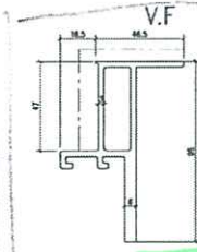
模號: X86292 名稱: GC頂橫 合金狀態: 6063-T6 重量: 2.301 KG/M V.F.: 213.3 mm
