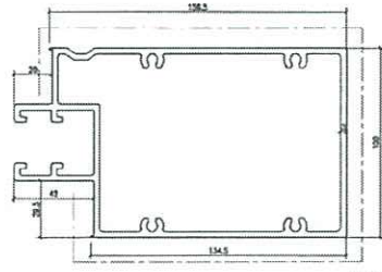
模號: X86302 名稱: 梗中橫 合金狀態: 6063-T6 重量: 5.428 KG/M V.F.: 125.4 mm
