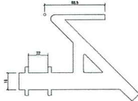
模號: X86256 名稱: 掛勾碼 合金狀態: 6061-T6 重量: 11.63 KG/M V.F.: - mm
