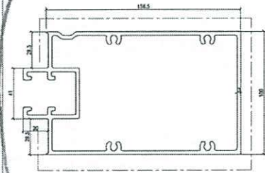
模號: X86308 名稱: Feature 中橫 合金狀態: 6063-T6 重量: 5.607 KG/M V.F.: 709.0 mm
