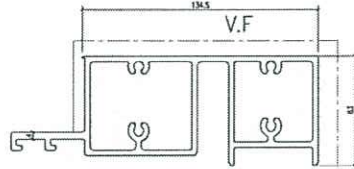
模號: X86280 名稱: 底橫 合金狀態: 6063-T6 重量: 5.134 KG/M V.F.: 381.0 mm
