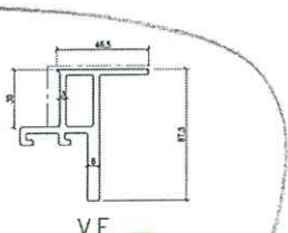
模號: X86291 名稱: GC中橫 合金狀態: 6063-T6 重量: 1.853 KG/M V.F.: 180.3 mm
