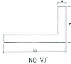
模號: X86257 名稱: 大鋁碼 合金狀態: 6061-T6 重量: 7.63 KG/M V.F.: - mm
