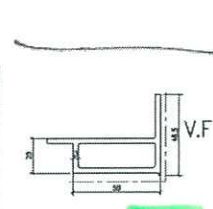
模號: X86290 名稱: GC企 合金狀態: 6063-T6 重量: 1.372 KG/M V.F.: 132.5 mm
