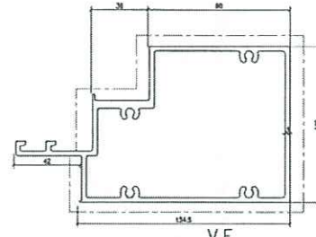
模號: X86281 名稱: 生下梗中橫 合金狀態: 6063-T6 重量: 4.926 KG/M V.F.: 489.9 mm
