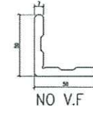
模號: X86318 名稱: 幕牆窗玉角 合金狀態: 6063-T5 重量: 1.624 KG/M V.F.: - mm
