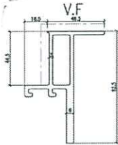
模號: X86293 名稱: GC底橫 合金狀態: 6063-T6 重量: 2.260 KG/M V.F.: 210.3 mm
