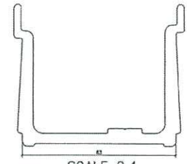
SCALE 2:1 NO V.F. 模號: X86303 名稱: 水槽芯 合金狀態: 6061-T6 重量: 2.329 KG/M V.F.: - mm
