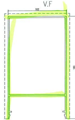
模號: X86320 名稱: 趟門中企室內收口框 合金狀態: 6063-T5 重量: 3.503 KG/M V.F.: 465.7 mm
