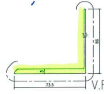
模號: X86460 名稱: 轉角面蓋 合金狀態: 6063-T5 重量: 1.226 KG/M V.F.: 147 mm
