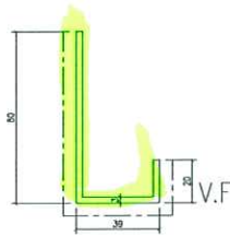
模號: X86463 名稱: 趟門陣底收口 合金狀態: 6063-T5 重量: 1.081 KG/M V.F.: 139.0 mm
