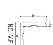
模號: X86318 名稱: 帶槽圓玉角 合金狀態: 6063-T5 重量: 1.624 KG/M V.F.: -
