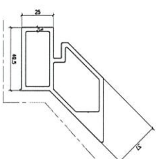
模號: X86310 名稱: 死牆轉角副框 合金狀態: 6063-T5 重量: 2.934 KG/M V.F.: 177.4 mm
