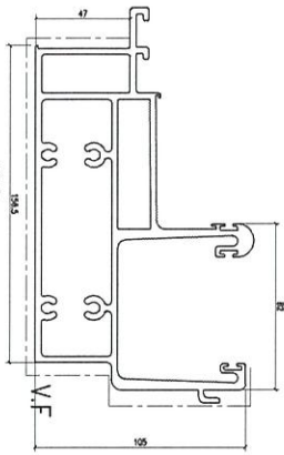
模號: X86279 名稱: 水槽樑 合金狀態: 6063-T6 重量: 7.453 KG/M V.F.: 538.0 mm
