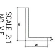
模號: X86287 名稱: 铝板角 合金狀態: 6063-T5 重量: 0.38 KG/M V.F.: -
