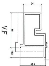
模號: X86313 名稱: 死牆生企副框 合金狀態: 6063-T5 重量: 2.079 KG/M V.F.: 179.9 mm
