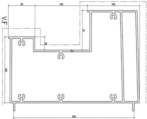
模號: X86307 名稱: Feature 合金狀態: 6063-T6 重量: 10.114KG/M V.F.: 657.2 mm
