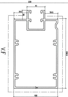
模號: X86308 名稱: Feature 中樑 合金狀態: 6063-T6 重量: 5.607 KG/M V.F.: 709.0 mm
