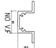
模號: X86319 名稱: 铝板加力骨 合金狀態: 6063-T5 重量: 1.389 KG/M V.F.: -
