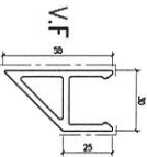
模號: X86286 名稱: 转角控河槽 合金狀態: 6063-T5 重量: 1.132 KG/M V.F.: 152.9 mm
