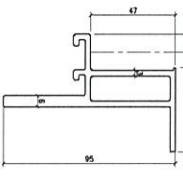
模號: X86292 名稱: GC頂橫 合金狀態: 6063-T6 重量: 2.301 KG/M V.F.: 213.3
