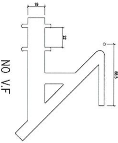
模號: X86256 名稱: 挂勾码 合金狀態: 6061-T6 重量: 11.63 KG/M V.F.: -
