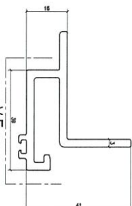
模號: X86305 名稱: 死牆梗 合金狀態: 6063-T5 重量: 0.988 KG/M V.F.: 80.7 mm
