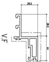
模號: X86299 名稱: 寶玉橫 合金狀態: 6063-T5 重量: 1.559 KG/M V.F.: 198.2 mm
