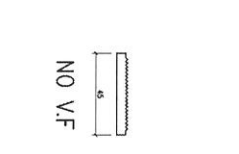
模號: X86260 名稱: 铝介子 合金狀態: 6061-T6 重量: 0.66 KG/M V.F.: -
