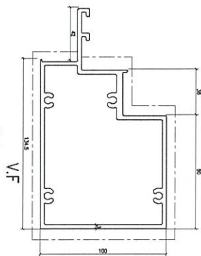
模號: X86281 名稱: 生下樑中樑 合金狀態: 6063-T6 重量: 4.926 KG/M V.F.: 489.9 mm
