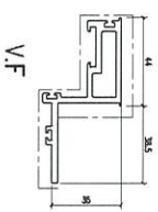
模號: X86285 名稱: 企鵝橫窗 合金狀態: 6063-T5 重量: 1.419 KG/M V.F.: 257.3 mm
