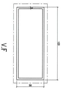
模號: X86298 名稱: 浴室橫料 合金狀態: 6063-T6 重量: 2.878 KG/M V.F.: 365.5 mm
