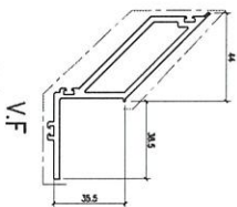
模號: X86297 名稱: 企转角生寶玉 合金狀態: 6063-T5 重量: 1.662 KG/M V.F.: 270.6 mm
