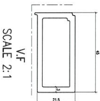
模號: X86305 名稱: 死牆梗 合金狀態: 6063-T5 重量: 0.988 KG/M V.F.: 80.7 mm
