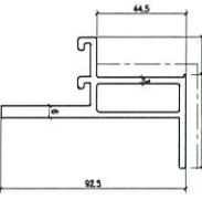
模號: X86293 名稱: GC底橫 合金狀態: 6063-T6 重量: 2.290 KG/M V.F.: 210.3
