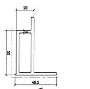
模號: X86290 名稱: GC企 合金狀態: 6063-T6 重量: 1.372 KG/M V.F.: 132.5
