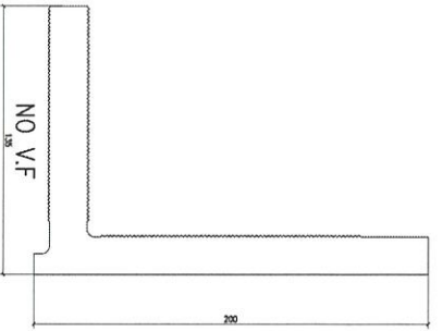
模號: X86254 名稱: 大铝码 合金狀態: 6061-T6 重量: 16.58 KG/M V.F.: -
