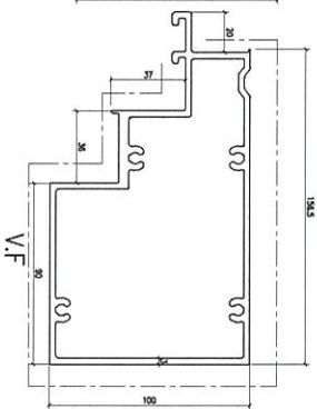
模號: X86309 名稱: 生中樑 合金狀態: 6063-T6 重量: 5.137 KG/M V.F.: 594.9 mm
