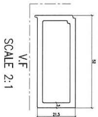
模號: X86304 名稱: 死牆轉角梗 合金狀態: 6063-T5 重量: 1.105 KG/M V.F.: 89.3 mm
