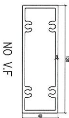
模號: X86289 名稱: 浴室中樑 合金狀態: 6063-T6 重量: 3.037 KG/M V.F.: - mm
