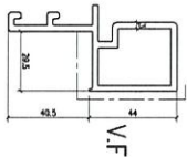
模號: X86312 名稱: 假企中橫 合金狀態: 6063-T5 重量: 1.742 KG/M V.F.: 184.5 mm
