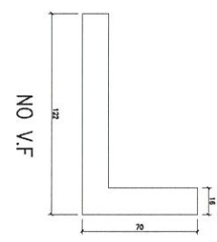
模號: X86257 名稱: 大铝码 合金狀態: 6061-T6 重量: 7.63 KG/M V.F.: -
