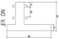
模號: X86255 名稱: 挂勾码 合金狀態: 6061-T6 重量: 6.63 KG/M V.F.: -
