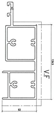
模號: X86280 名稱: 底樑 合金狀態: 6063-T6 重量: 5.134 KG/M V.F.: 381.0 mm
