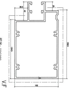
模號: X86302 名稱: 硬中樑 合金狀態: 6063-T6 重量: 5.428 KG/M V.F.: 425.4 mm
