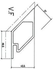
模號: X86311 名稱: 生下梗轉角副框 合金狀態: 6063-T5 重量: 2.219 KG/M V.F.: 151.0 mm
