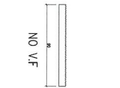
模號: X86259 名稱: 铝介子 合金狀態: 6061-T6 重量: 1.83 KG/M V.F.: -
