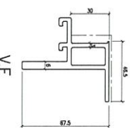
模號: X86291 名稱: GC中橫 合金狀態: 6063-T6 重量: 1.863 KG/M V.F.: 180.3
