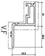
模號: X86284 名稱: 企生寶玉 合金狀態: 6063-T5 重量: 1.443 KG/M V.F.: 263.3 mm
