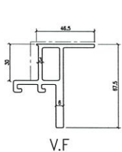
模號: X86291 名稱: GC中橫 合金狀態: 6063-T6 重量: 1.853 KG/M V.F.: 180.3 mm
