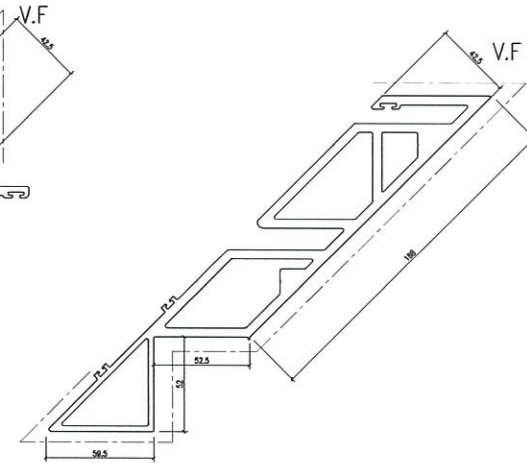
模號: X86296 名稱: 转角梗母企 合金狀態: 6063-T6 重量: 10.321 KG/M V.F.: 553.4 mm
