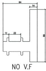
模號: X86255 名稱: 掛勾碼 合金狀態: 6061-T6 重量: 6.63 KG/M V.F.: - mm
