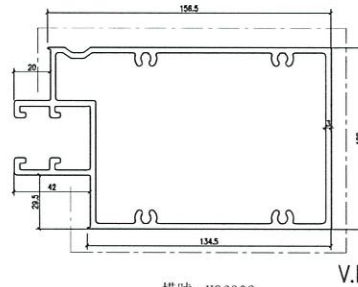
模號: X86302 名稱: 梗中橫 合金狀態: 6063-T6 重量: 5.428 KG/M V.F.: 425.4 mm
