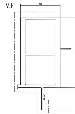
模號: X86278 名稱: 梗邊企 合金狀態: 6063-T6 重量: 9.065 KG/M V.F.: 340.6 mm
