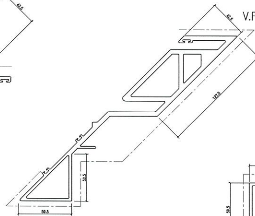
模號: X86276 名稱: 转角生母企 合金狀態: 6063-T6 重量: 8.759 KG/M V.F.: 575.1 mm
