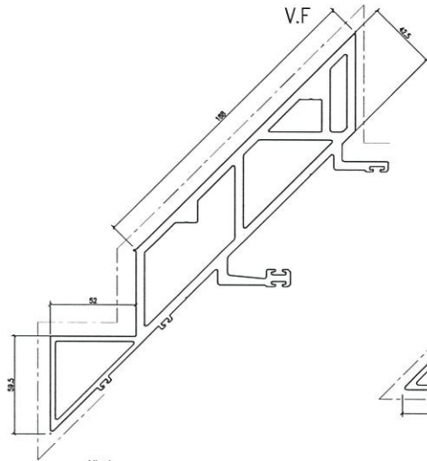
模號: X86275 名稱: 转角梗公企 合金狀態: 6063-T6 重量: 11.491 KG/M V.F.: 558.1 mm
