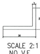
模號: X86287 名稱: 鋁板角 合金狀態: 6063-T5 重量: 0.38 KG/M V.F.: - mm
