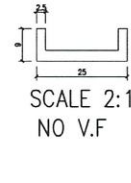
模號: X86258 名稱: 鋁介子 合金狀態: 6061-T6 重量: 0.28 KG/M V.F.: - mm
