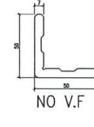
模號: X86318 名稱: 幕牆窗玉角 合金狀態: 6063-T5 重量: 1.624 KG/M V.F.: - mm
