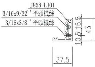
SECTION D-D
