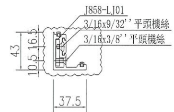
SECTION D-D
