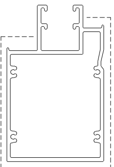
模號: X86061 名稱: 瘦窗中橫 合金狀態: 6063-T6 重量: 6.483 KG/M V.F.: 0.4265 m 2 /m
