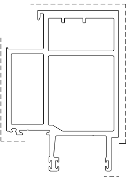
模號: X86057 名稱: 公企料 合金狀態: 6063-T6 重量: 10.577KG/M V.F.: 0.4810 m 2 /m
