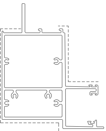
模號: X86070 名稱: 頂橫料 合金狀態: 6063-T5 重量: 10.370KG/M V.F.: 0.6084 m 2 /m
