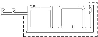
模號: X86049 名稱: 母企料 合金狀態: 6063-T6 重量: 6.724 KG/M V.F.: 0.3934 m 2 /m
