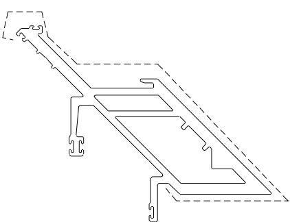
模號: X86051 名稱: 公企料(轉角) 合金狀態: 6063-T6 重量: 9.711 KG/M V.F.: 0.4678 m 2 /m
