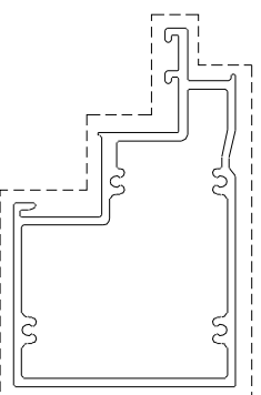
模號: X86063 名稱: 生窗中橫 合金狀態: 6063-T6 重量: 5.960 KG/M V.F.: 0.5189 m 2 /m
