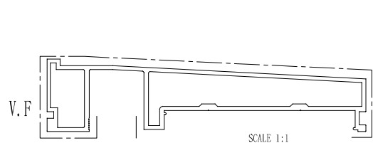
模號: X86355 名稱: 攔河頂橫料 合金狀態: 6063-T6 重量: 5.573 KG/M V.F.: 539.3 mm
