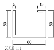
模號: X86356 名稱: 攔河底托料 合金狀態: 6063-T6 重量: 2.114 KG/M V.F.: 0 mm
