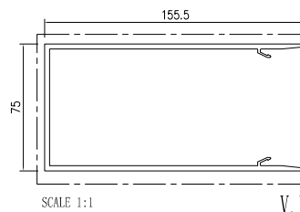
模號: X86357 名稱: 後蓋 (企向) 合金狀態: 6063-T6 重量: 3.088 KG/M V.F.: 389 mm
