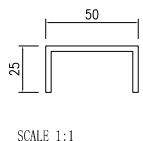
模號: A575 名稱: 前拍蓋底托料 合金狀態: 6063-T6 重量: 0.761 KG/M V.F.: 0 mm
