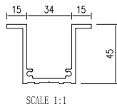
模號: 名稱: 加力骨 合金狀態: 6063-T6 重量: 1.318 KG/M V.F.: 0 mm
