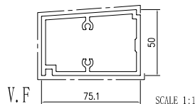
模號: 名稱: 裝飾條1 合金狀態: 6063-T6 重量: 2.181 KG/M V.F.: 205.4 mm
