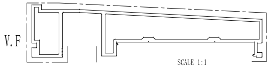
模號: X86355 名稱: 攔河頂橫料 合金狀態: 6063-T6 重量: 5.573 KG/M V.F.: 539.3 mm
