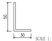
模號: N579 名稱: 50x30x3鋁角 合金狀態: 6063-T6 重量: 0.583 KG/M V.F.: 0 m 2 /m
