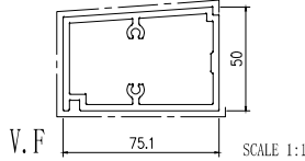
模號: X86103 名稱: 裝飾條1 合金狀態: 6063-T6 重量: 2.181 KG/M V.F.: 205.4 mm
