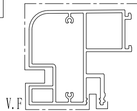
模號: X86105 名稱: 小裝飾條(橫2) 合金狀態: 6063-T6 重量: 4.837 KG/M V.F.: 0.3488 m 2 /m
