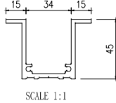
模號: X86146 名稱: 加力骨 合金狀態: 6063-T6 重量: 1.318 KG/M V.F.: 0 mm
