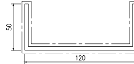
模號: H118688 名稱: 120x50x4mm厚鋁槽 合金狀態: 6063-T6 重量: 2.289 KG/M V.F.: 0.448 m 2 /m
