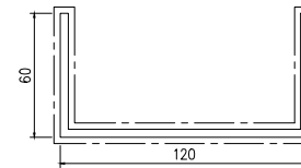
模號: A00929 名稱: 120x60x4mm厚鋁槽 合金狀態: 6063-T6 重量: 2.505 KG/M V.F.: 0.488 m 2 /m
