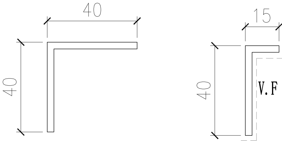
用40*40*3铝角切成40*35铝槽然后喷油
