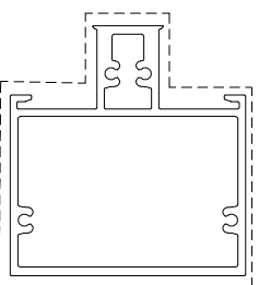
模號: X86069 名稱: 生窗中橫 合金狀態: 6063-T6 重量: 5.621 KG/M V.F.: 0.5117 m 2 /m
