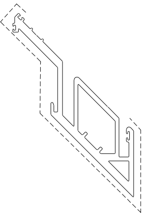
模號: X86052 名稱: 母企料(轉角) 合金狀態: 6063-T6 重量: 7.942 KG/M V.F.: 0.4441 m 2 /m
