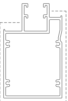
模號: X86061 名稱: 榎窗中橫 合金狀態: 6063-T6 重量: 6.483 KG/M V.F.: 0.4265 m 2 /m
