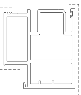
模號: X86058 名稱: 母企料 (生窗) 合金狀態: 6063-T6 重量: 10.159KG/M V.F.: 0.4375 m 2 /m
