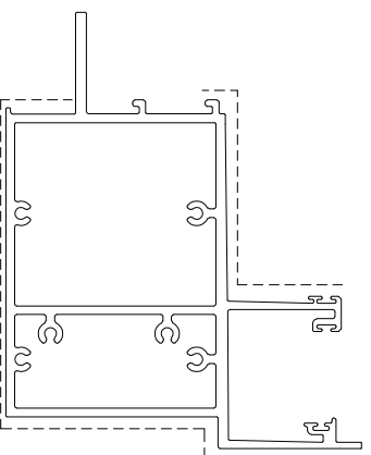
模號: X86066 名稱: 生窗中橫 合金狀態: 6063-T6 重量: 8.652 KG/M V.F.: 0.5865 m 2 /m
