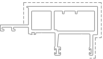
模號: X86047 名稱: 公企料 合金狀態: 6063-T6 重量: 7.516 KG/M V.F.: 0.4086 m 2 /m
