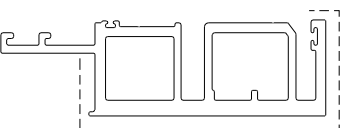
模號: X86049 名稱: 母企料 合金狀態: 6063-T6 重量: 6.724 KG/M V.F.: 0.3934 m 2 /m
