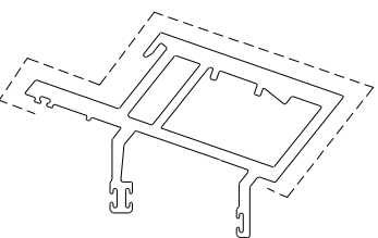
模號: X86053 名稱: 公企料(轉角) 合金狀態: 6063-T6 重量: 6.761 KG/M V.F.: 0.3565 m 2 /m
