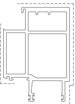
模號: X86057 名稱: 公企料 合金狀態: 6063-T6 重量: 10.577KG/M V.F.: 0.4810 m 2 /m
