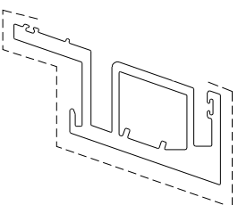
模號: X86054 名稱: 母企料(轉角) 合金狀態: 6063-T6 重量: 5.713 KG/M V.F.: 0.3371 m 2 /m
