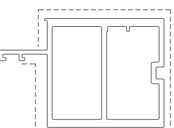
模號: X86056 名稱: 中企料 合金狀態: 6063-T6 重量: 9.903 KG/M V.F.: 0.4975 m 2 /m
