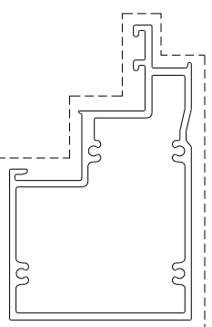
模號: X86063 名稱: 生窗中橫 合金狀態: 6063-T6 重量: 5.960 KG/M V.F.: 0.5189 m 2 /m
