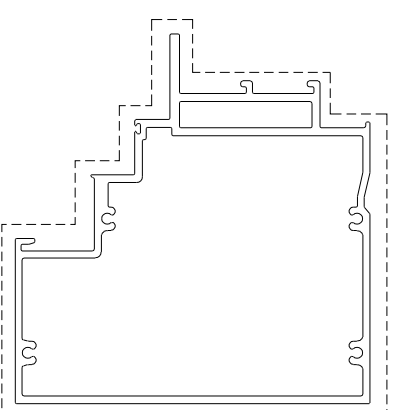
模號: X86063 名稱: 生窗中橫 合金狀態: 6063-T6 重量: 5.960 KG/M V.F.: 0.5189 m 2 /m
