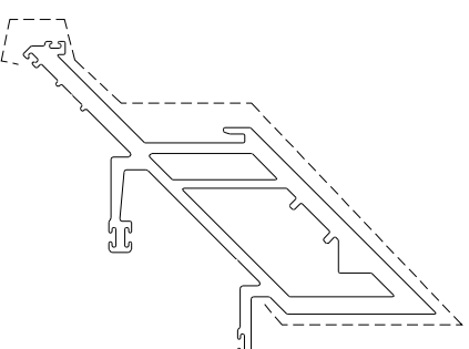
模號: X86051 名稱: 公企料(轉角) 合金狀態: 6063-T6 重量: 9.711 KG/M V.F.: 0.4678 m 2 /m
